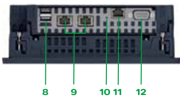
Premium型控制模块底视图
