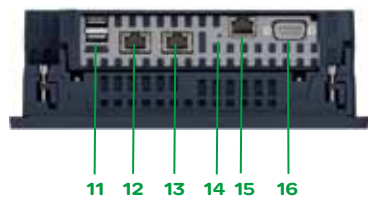
Open型控制模块的底视图
